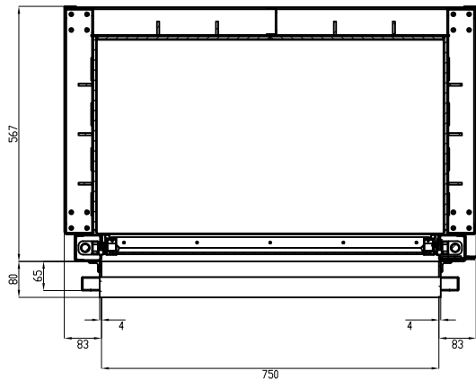
SEZIONE B-B
